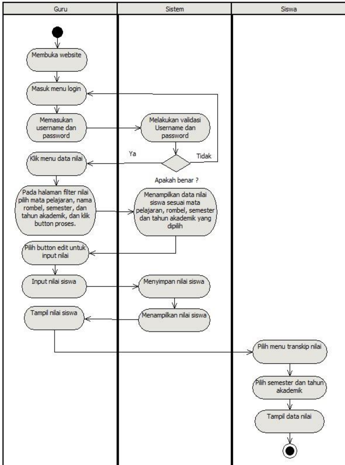
Gambar 5. Activity Diagram Sistem Informasi Kelola Nilai
